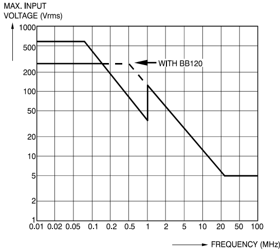
그림 10. 최대 입력 전압 대 주파수
