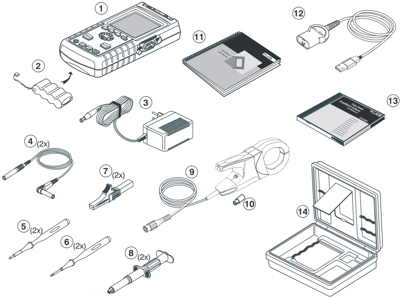
그림 1. 휴대 케이스 내용물
