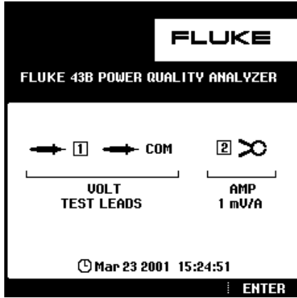
그림 3. 시작 화면
