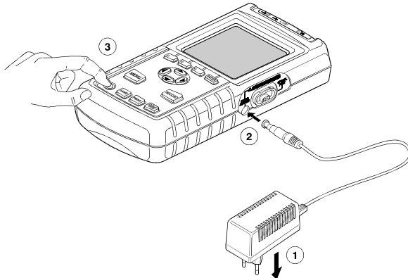
그림 2. Fluke 43B 에 대한 전원의 연결
